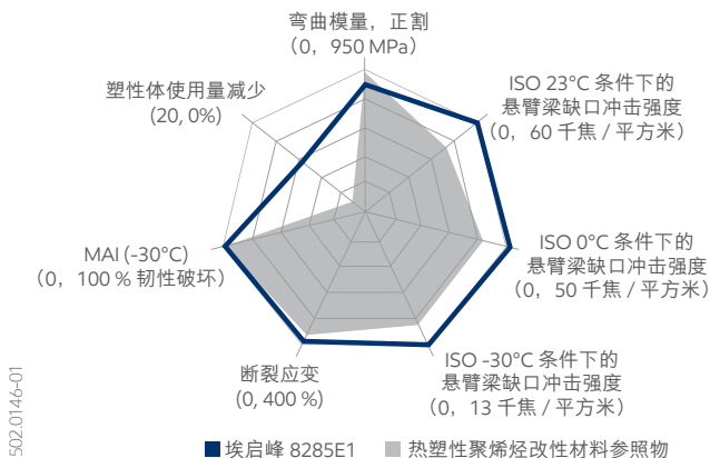
图 2： 含埃启峰 8285E1 的改性材料与传统抗冲共聚聚丙烯 (ICP) 改性材料参照物的性能数据对比。塑性体使用量从热塑性聚烯烃改性材料参照物中的 20% 减少为埃启峰 8285E1 改性材料中的 10%。
